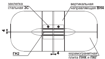
Схема установки панелей из натурального камня и агломерата на клипсы из элемента крепления ГН2
