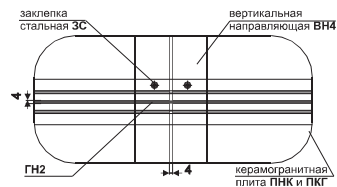
Схема установки панелей из натурального камня и агломерата на элемент крепления ГН2
