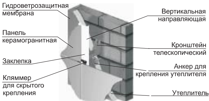
Рис. 1. Основные элементы конструкции системы МК4-01
