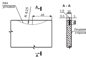
Обработка панели керамогранитной под клипсы КТС, ККС
