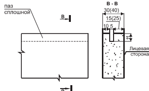
Обработка панели из натурального камня и агломерата под элемент крепления ГН2
