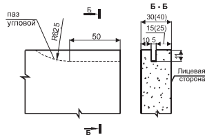
Обработка панели из натурального камня и агломерата под клипсы из элемента крепления ГН2
