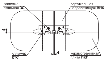
Схема установки панелей керамогранитных на клипсах
