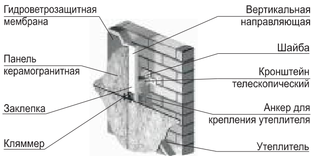
Рис. 1. Основные элементы конструкции системы МК2-01
