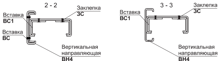
Узел начала облицовки.
